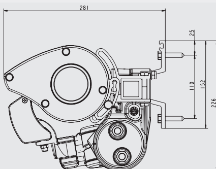
Nova kassett väggmontering
