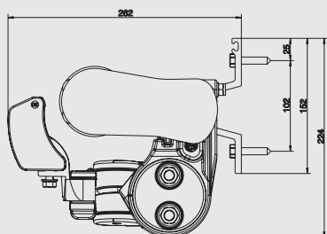
Nova classic väggmontering
