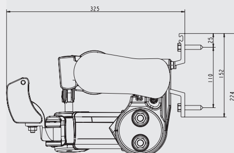
Nova Marcesa väggmontering
