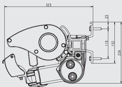
Nova Marcesa kassett väggmontering
