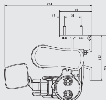
Nova rullgardinsfront vägg/takmontering
