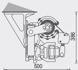
Takmontering
